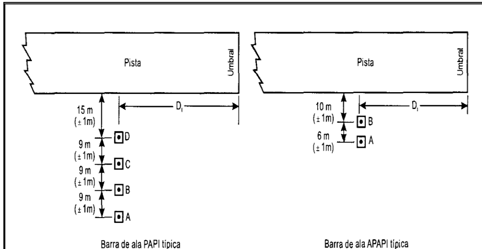
Figura 5-18. Emplazamiento del PAPI y del APAPI
