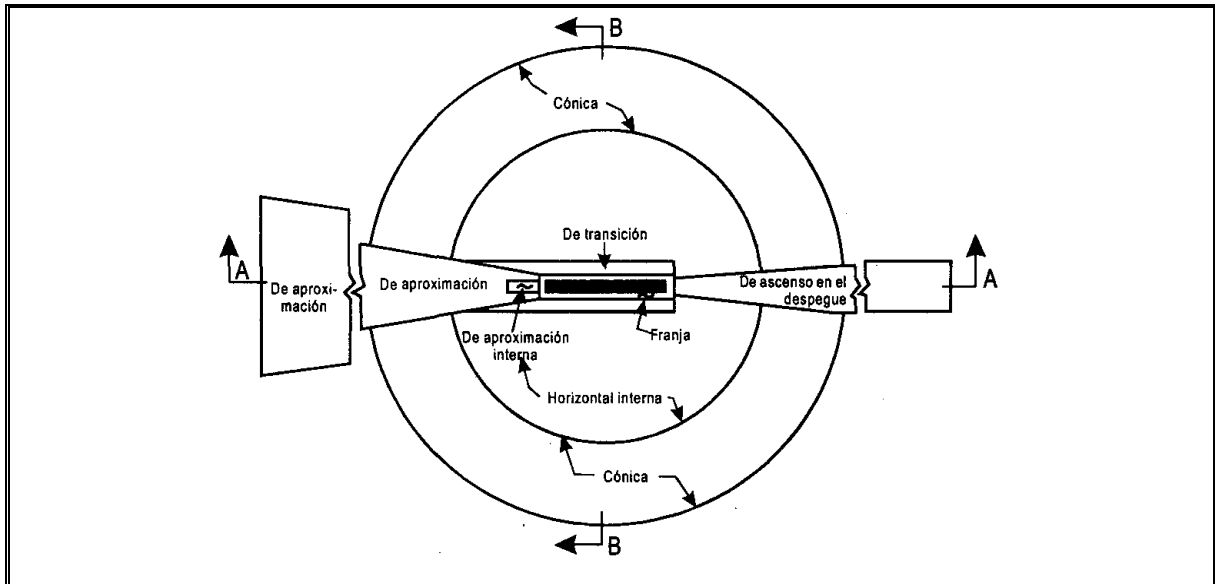
Figura 4 - 1. Superficies limitadoras de obstáculos
