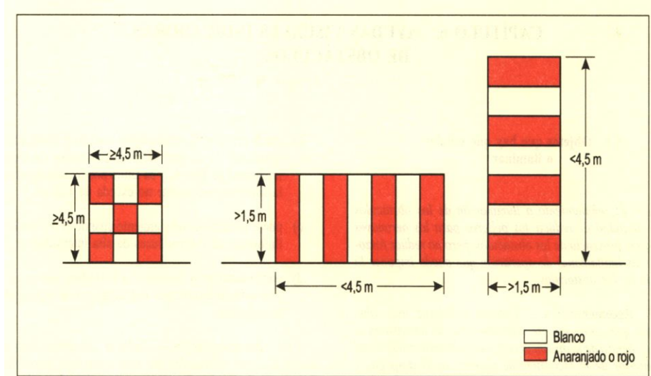
Figura 6-1. Configuración básica del señalamiento de obstáculos
